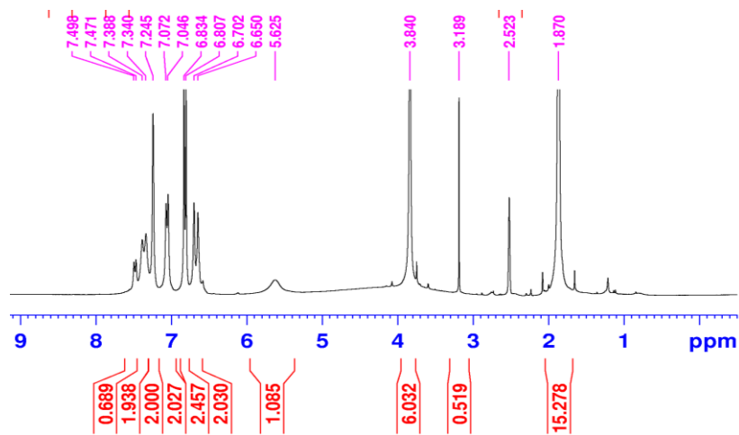
شکل ۷. طیف ^1\text{H NMR} نانو کمپلکس [\text{Zn}(\text{Cur})_2(\text{H}_2\text{O})_2] (1)
