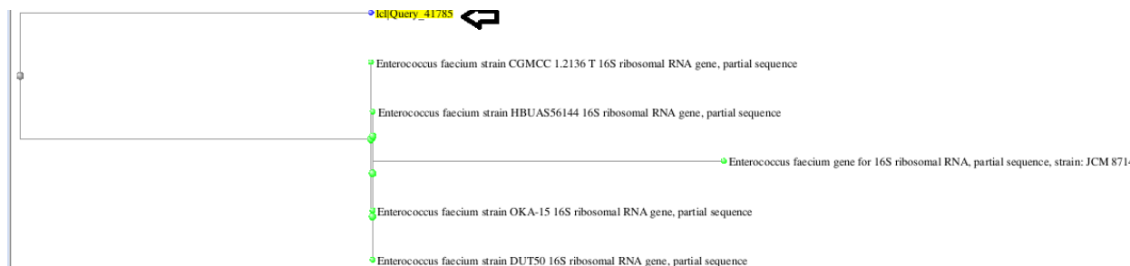
شکل ۵: درخت فیلوژنی به دست آمده از سایت NCBI در مورد نمونه باکتری ۳. این دندروگرام از نظر توالی این بخش از ژن ۱۶S rRNA نشاندهنده واریانت جدیدی می‌باشد.
