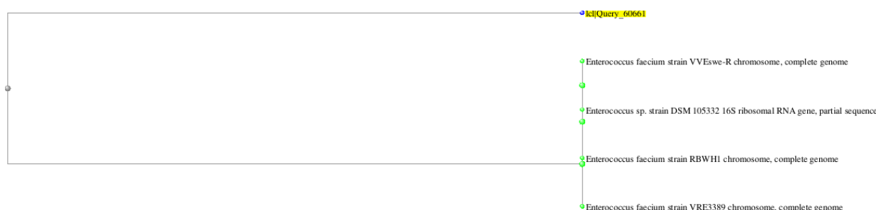
شکل ۷: درخت فیلوژنی بدست آمده از سایت NCBI در مورد نمونه باکتری ۱۳. این دندروگرام از نظر توالی این بخش از ژن ۱۶S rRNA نشاندهنده واریانت جدیدی می‌باشد.
