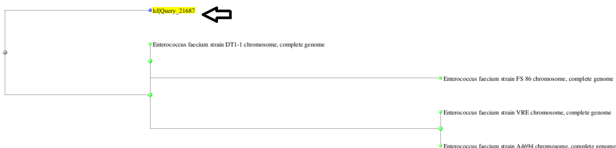
شکل ۶: درخت فیلوژنی به دست آمده از سایت NCBI در مورد نمونه باکتری ۸. این دندروگرام از نظر توالی این بخش از ژن ۱۶S rRNA نشاندهنده واریانت جدیدی می‌باشد.
