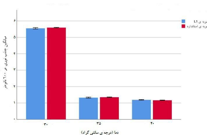
شکل ۴. رشد سویه ی L1 و سویه ی استاندارد PTCC: 1330 در دماهای مختلف ( P < 0.05 )
