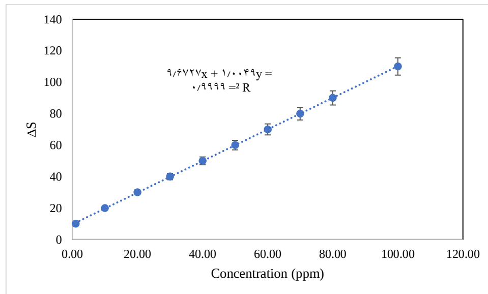
شکل ۵- منحنی کالیبراسیون
